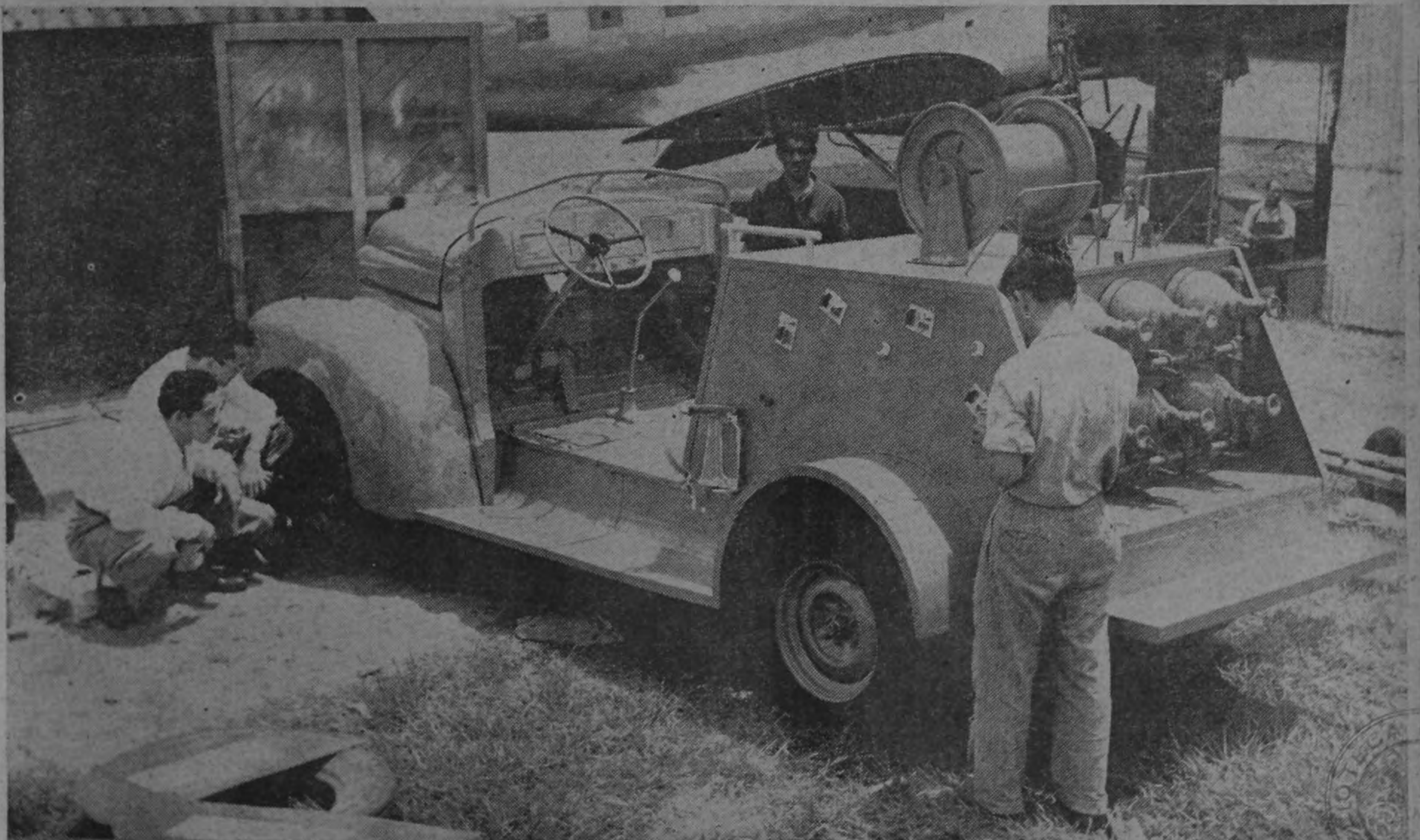
BOMBA NACIONAL. — Esta pequeña Bomba de Incendios fué construída en los talleres de SALA, con la cooperación de todos los jefes y empleados. Está acondicionada con extinguidores potentes y especiales, para casos de emergencia. Otra prueba de la eficacia e ingenio del trabajador costarricense. — (Foto CARRILLO)
